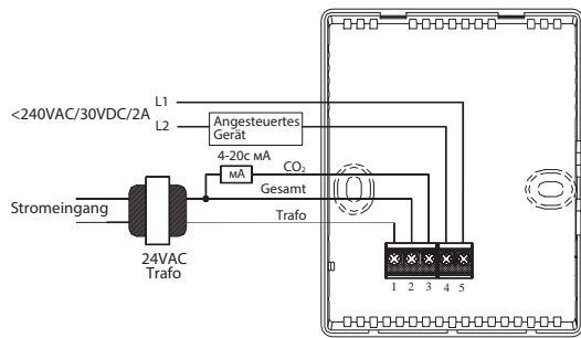
Abb. 4. Anschlussschema
