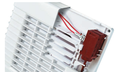
Stromversorgung des Gitters EIN – Lamellenverschlüsse OFFEN
