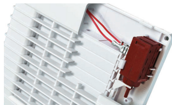
Stromversorgung des Gitters AUS – Lamellenverschlüsse GESCHLOSSEN
